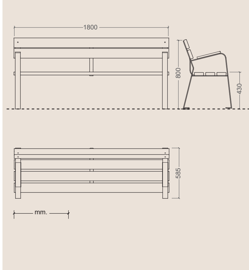
BANCO ALAMEDA (CON PROTECTORES APOYABRAZOS) BENCH "ALAMEDA" (WITH PROTECTED ARMSETS) BANC "ALAMEDA" (AVEC PROTECTEURS APPUIE-BRAS)
