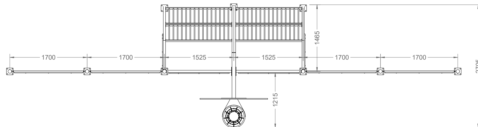
Planta
