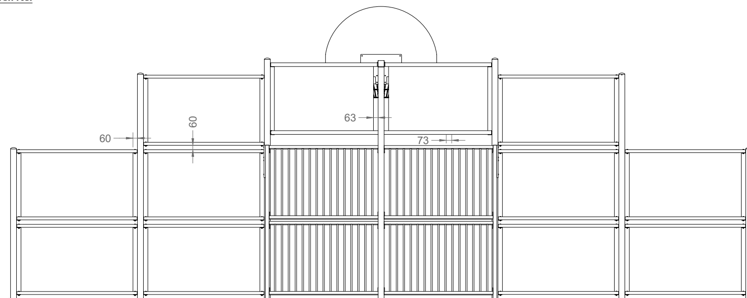
Alzado Posterior
