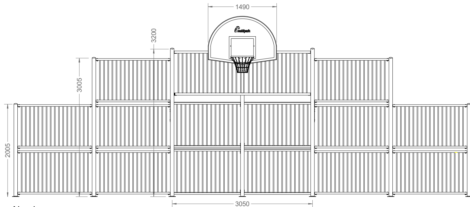
Alzado
