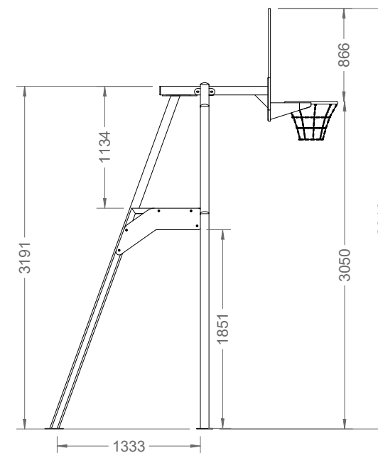
Perfil
