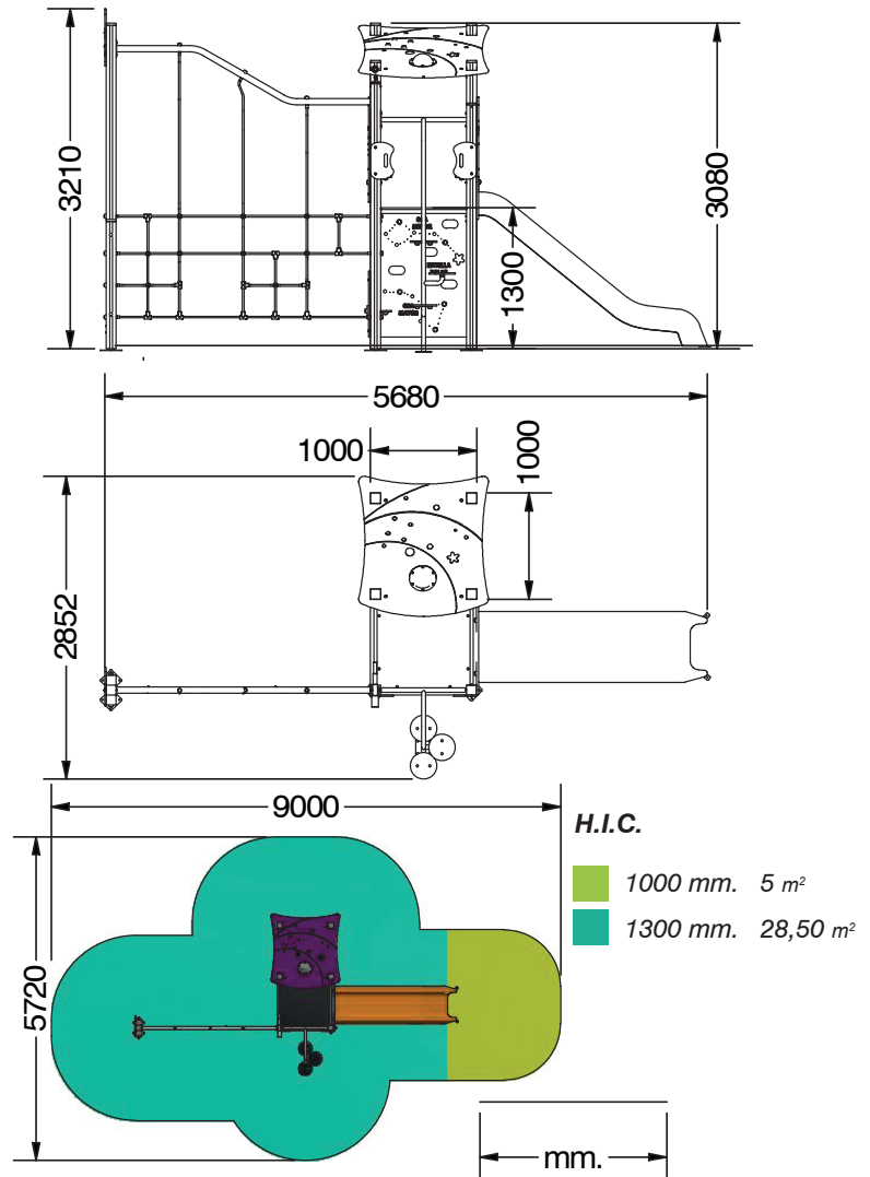
"NOVA" (MADERA) CON TREPA "NOVA" (WOODEN) WITH CLIMBING FRAME "NOVA" (EN BOIS) AVEC FILET À GRIMPER
